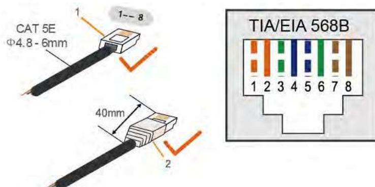
1: Fiche RJ45
