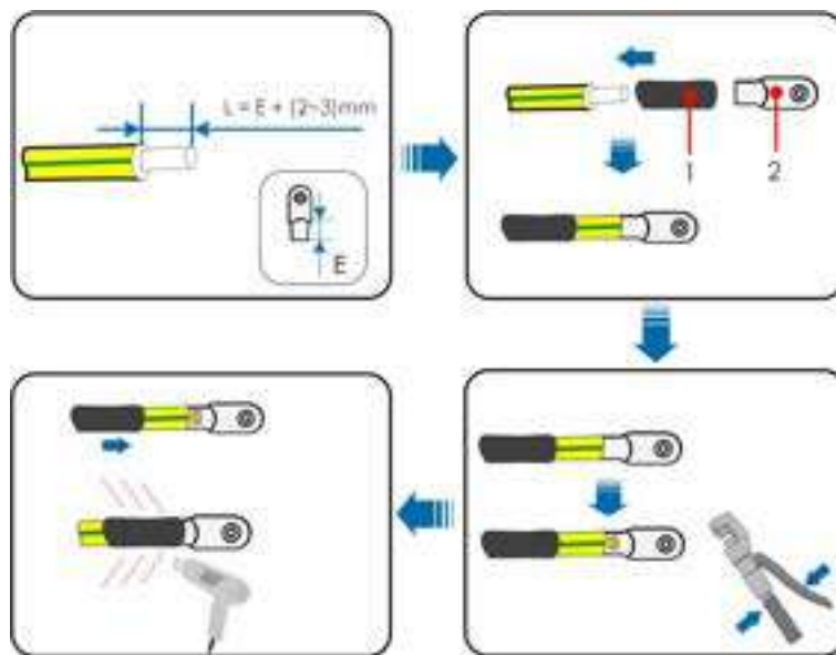
(1) Gaine thermorétractable
