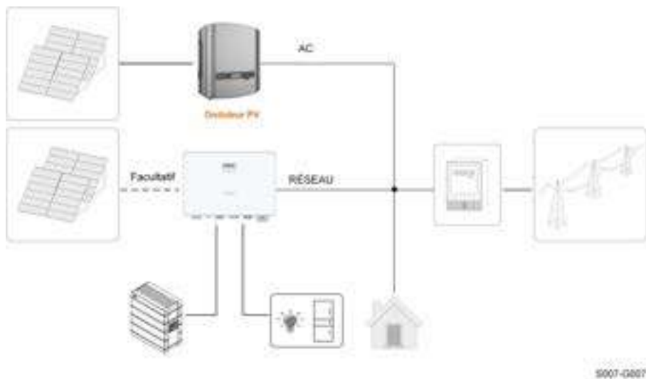
figure 2-6 Adaptation de(s) onduleur(s) PV existant(s) au port de l'onduleur hybride sur le réseau
