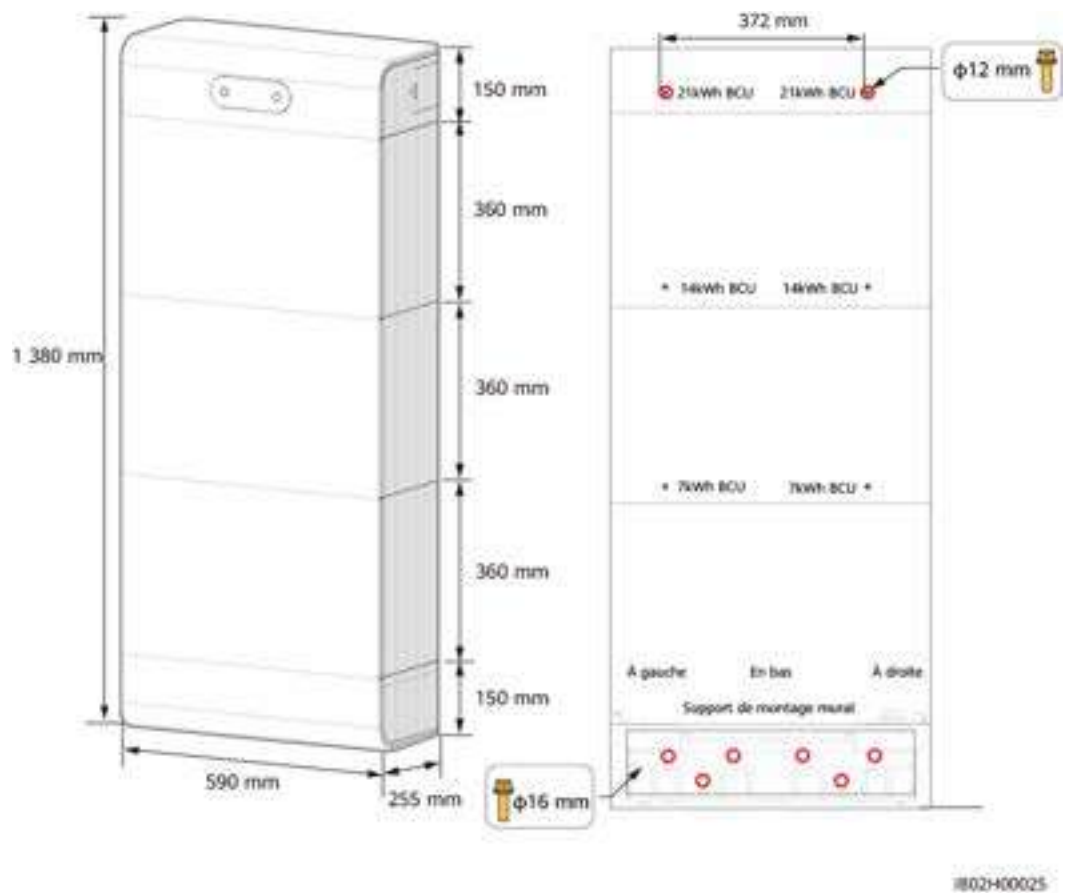
Figure 4-5 Dimensions pour le montage mural
