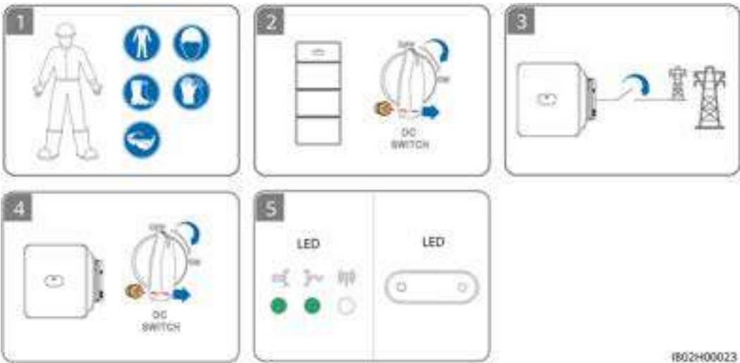
Figure 6-1 Processus d'allumage
