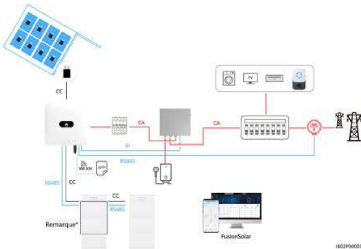
Figure 2-8 Scénario sur/hors réseau
